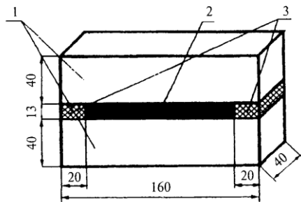
Рисунок 2 – Образец деформационного шва
