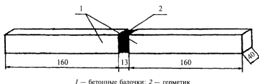
Рисунок 4 – Образец деформационного шва для определения показателя выносливости
